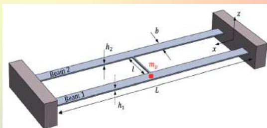
Конструкция чувствительного элемента микромеханического детектора масс сверхмалых осажждённых частиц
