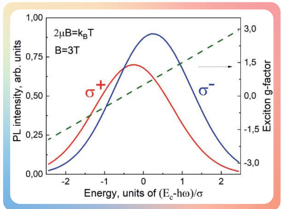
Спектры излучения ансамбля экситонов в круговых поляризациях \sigma^+ и \sigma^- в магнитном поле B = 3 T в зависимости от безразмерной энергии \epsilon/\sigma при сильной спиновой релаксации и в предположении, что g-фактор линейно зависит от энергии экситона и меняет знак в пределах полосы ФЛ
