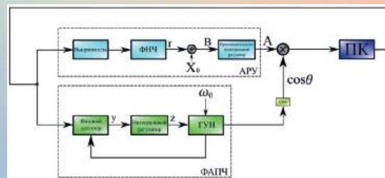
Схема генерации стационарных колебаний микроэлектромеханического резонатора
